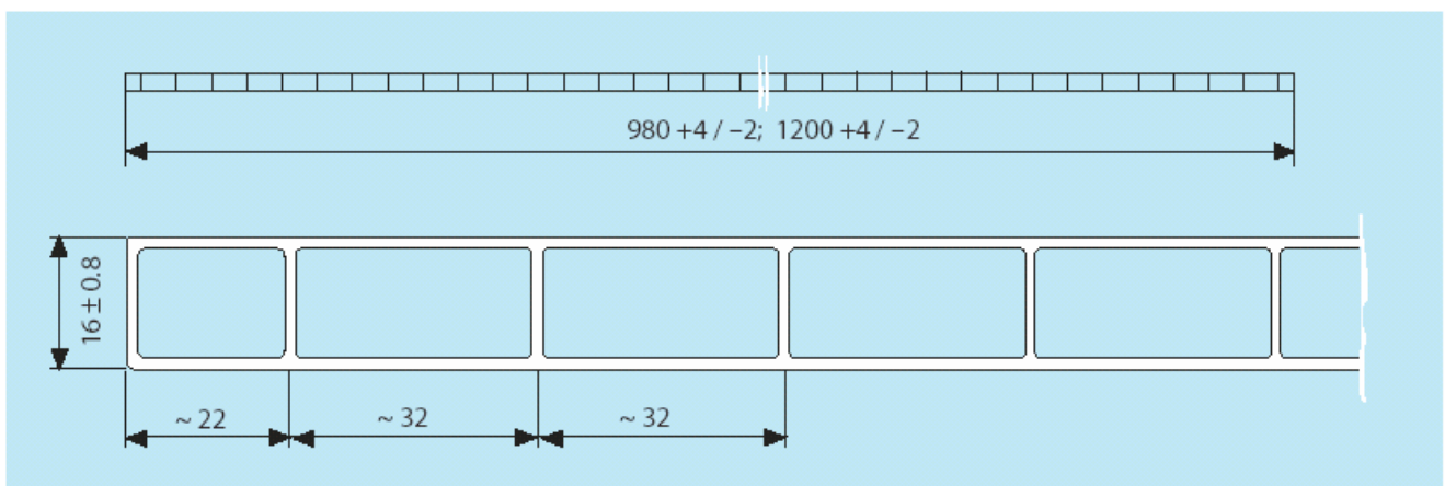
Сечение: PLEXIGLAS HEATSTOP® SDP 16 (Размеры в мм)
